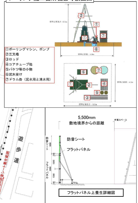
ボーリング施工箇所機器等設置図
