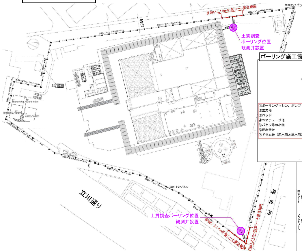
作業場所計画図
