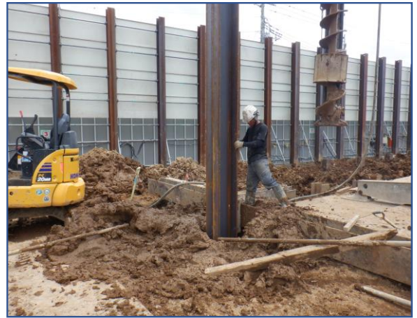
山留設置
